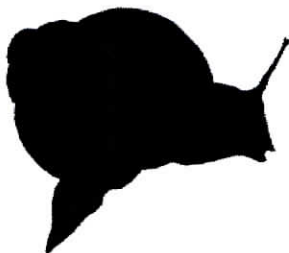
2. Дақты шешім
