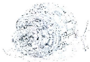
1. Сызықтық шешім
