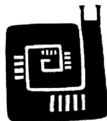
4. Геометриялық шешім
